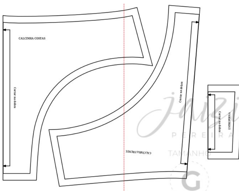
Figura 1- Visão geral do molde
